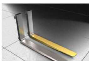
HORQUILLAS EN COBRE O ACERO INOXIDABLE Espesor cobertura: 4 mm Aplicación de una fuerte protección
